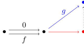
Abbildung 9: Das Kommutative Diagramm für einen Kokern
