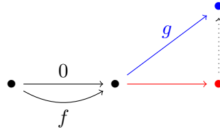
Abbildung 9: Das Kommutative Diagramm für einen Kokern
