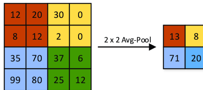
Abbildung 25: Average Pooling mit 2 \times 2 großen Submatritzen
