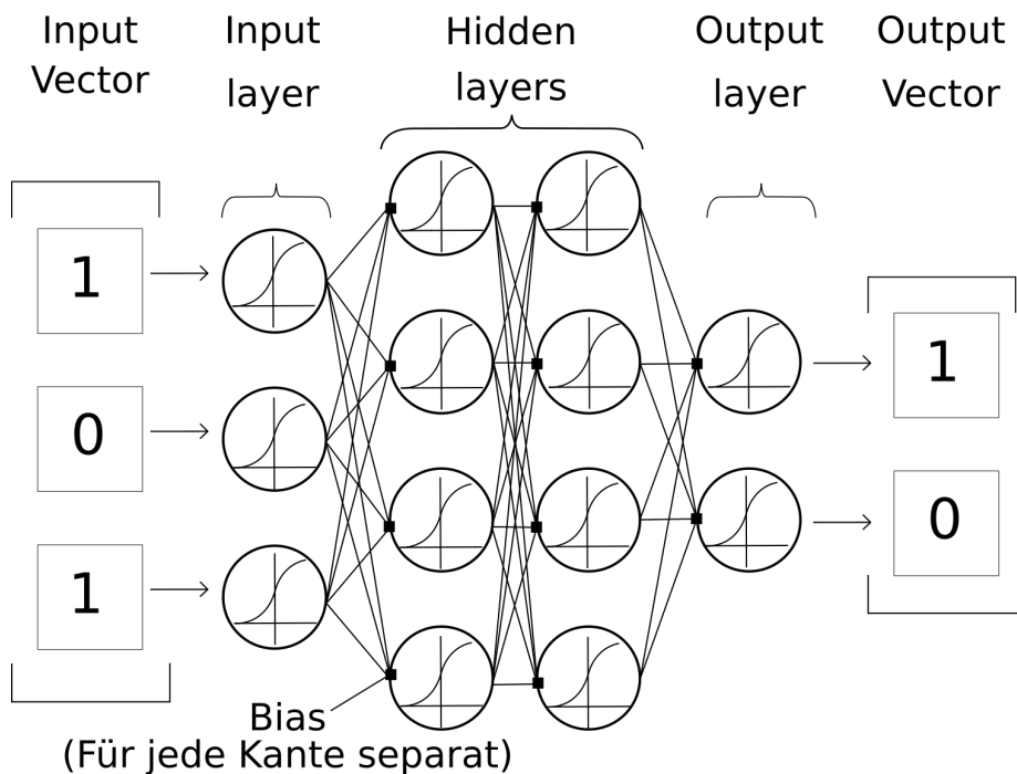
Abbildung 2: Ein einfaches neuronales Netz
